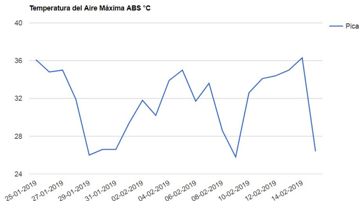
Figura 2.- Temperaturas Maximas
